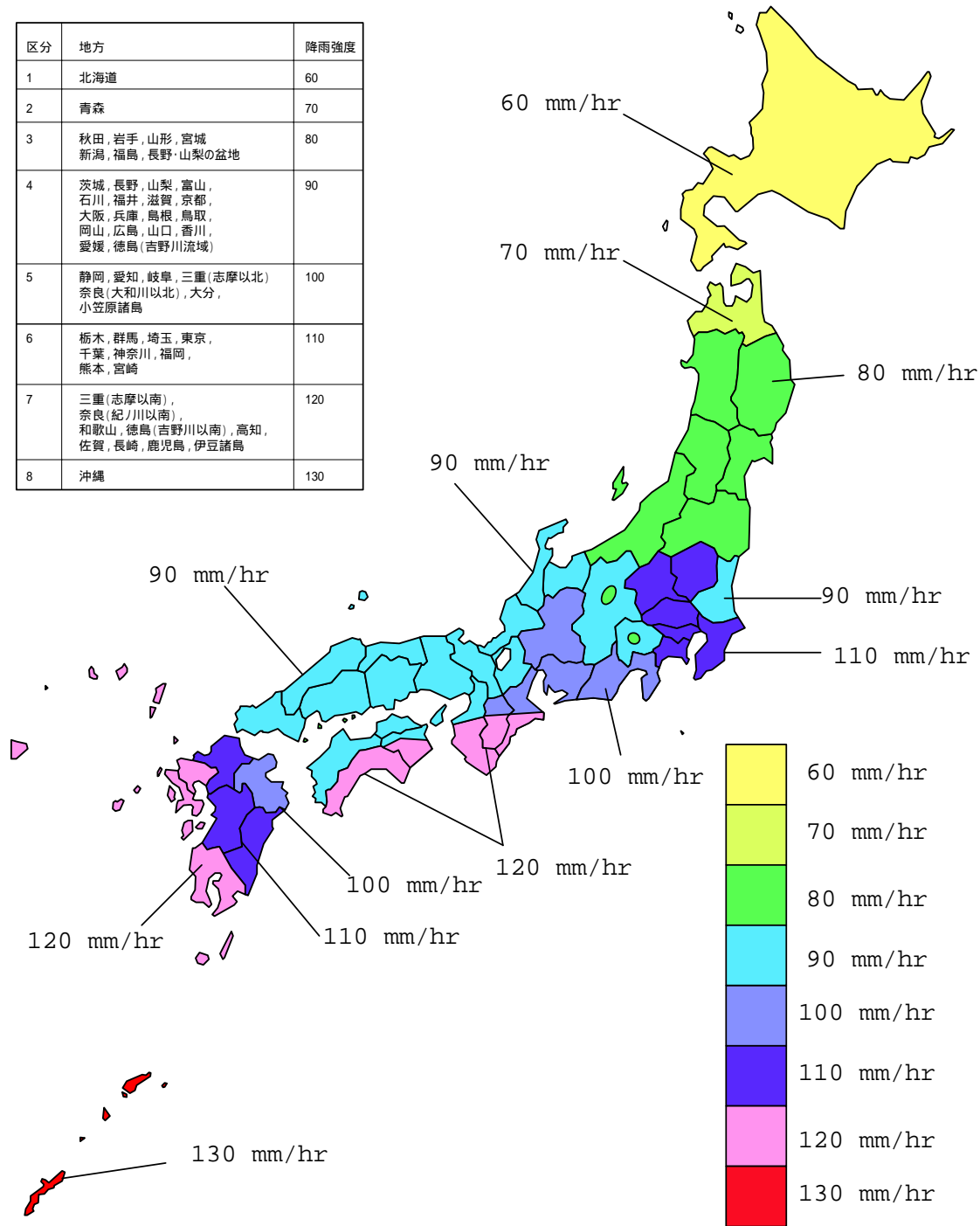
解図 2 - 14 路面排水工等に用いる標準降雨強度 (3年確率10分間降雨強度)
