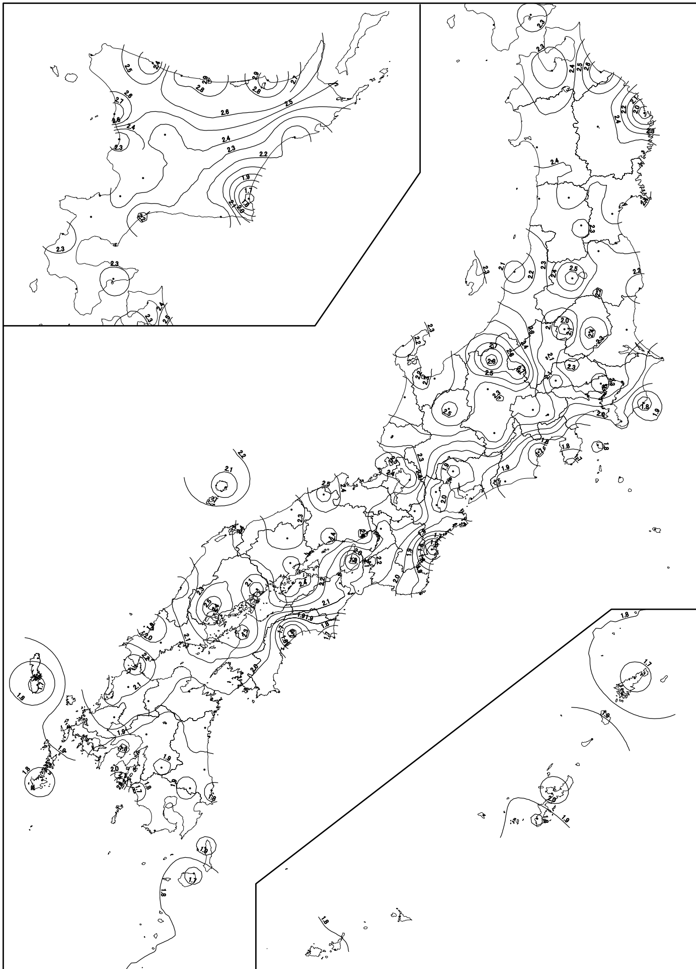
\beta 分布图
