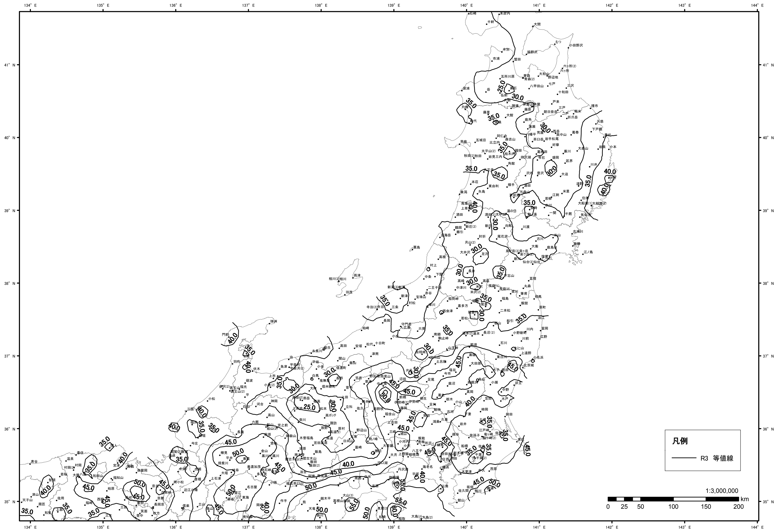
図 3年確率アメダス時間雨量 (R3) — 東北～関東～北陸
