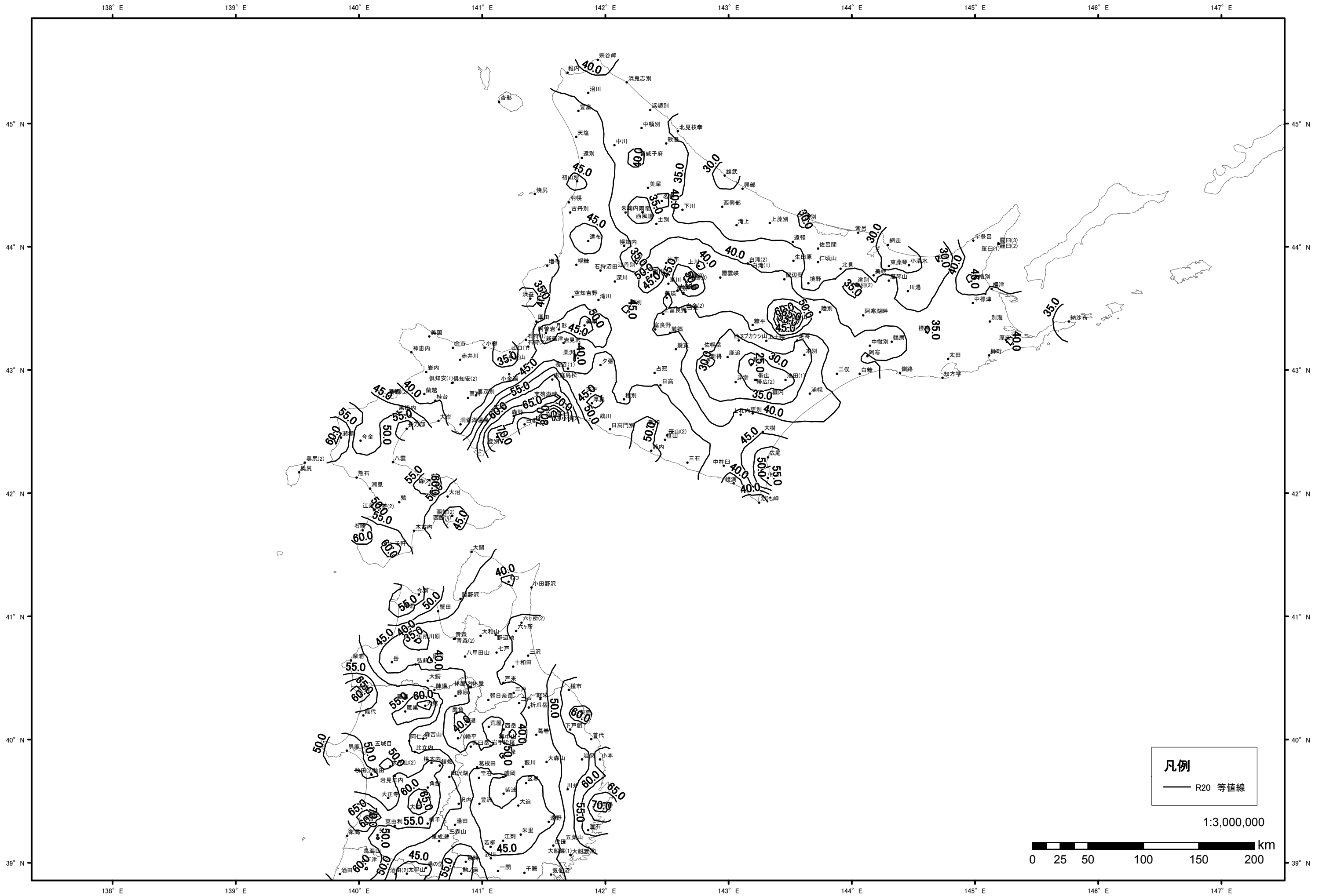
図 20年確率アメダス時間雨量 (R20) — 北海道～北東北
