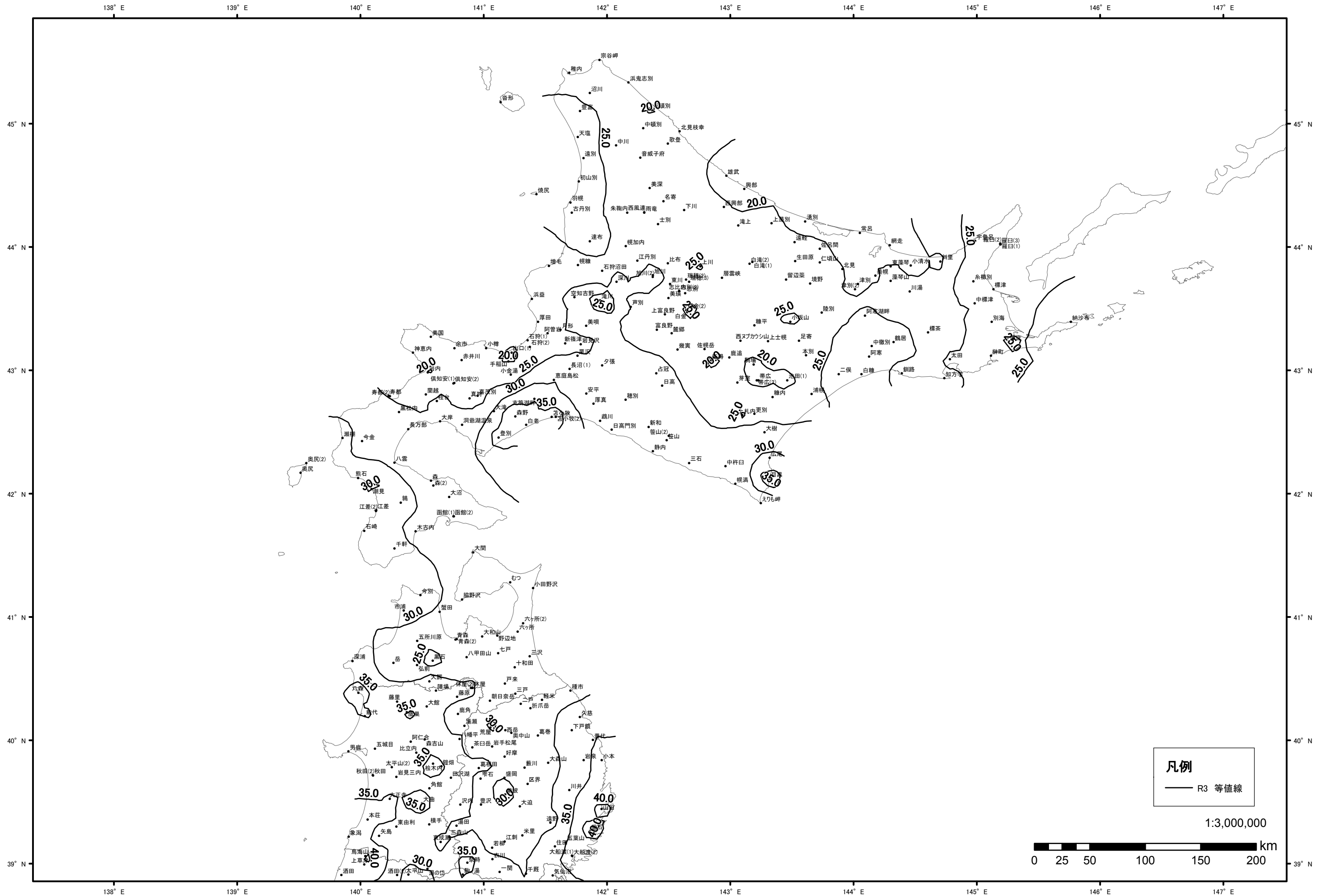
3年確率アメダス時間雨量 (R3) — 北海道～北東北
