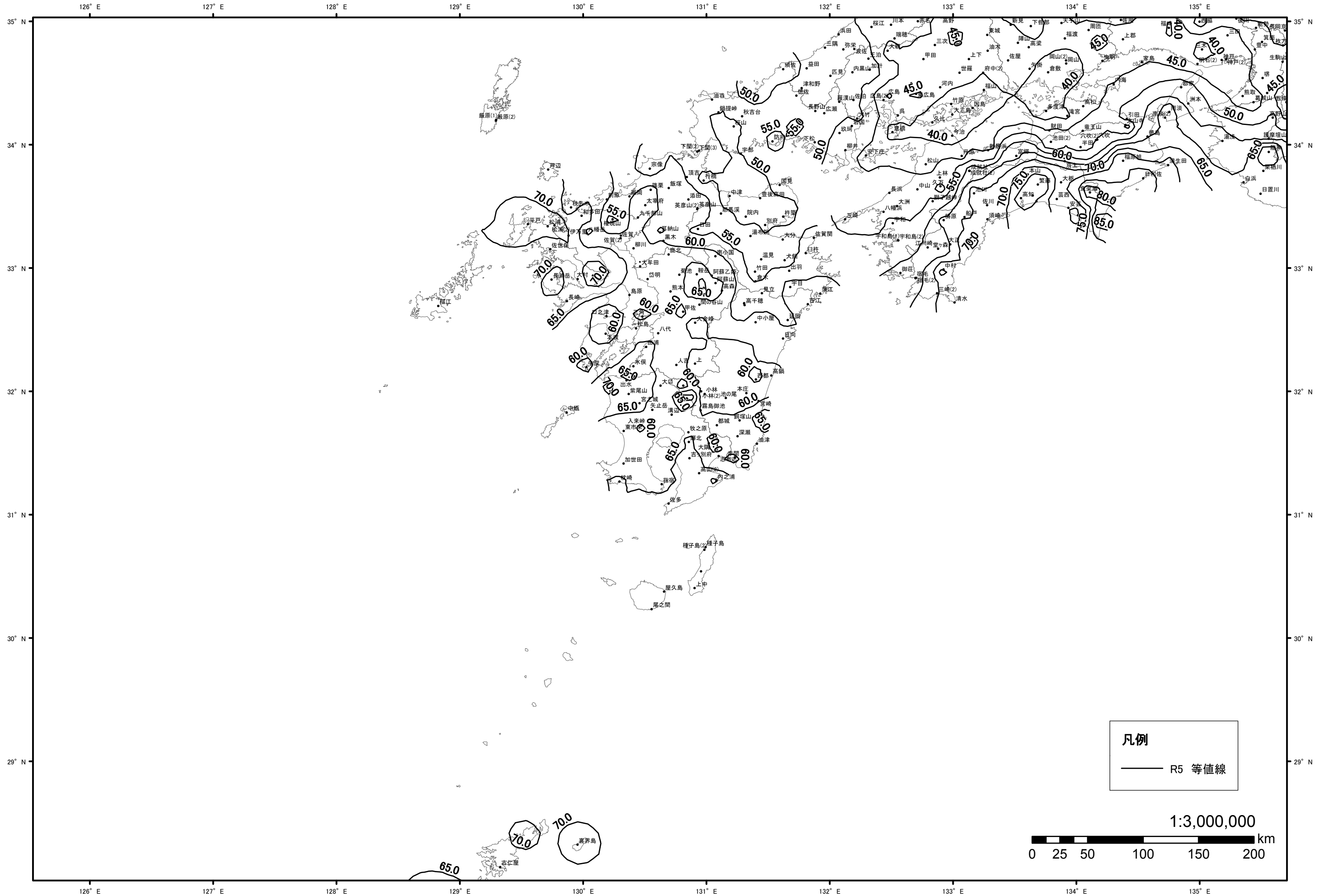
5年確率アメダス時間雨量 (R5) — 九州
