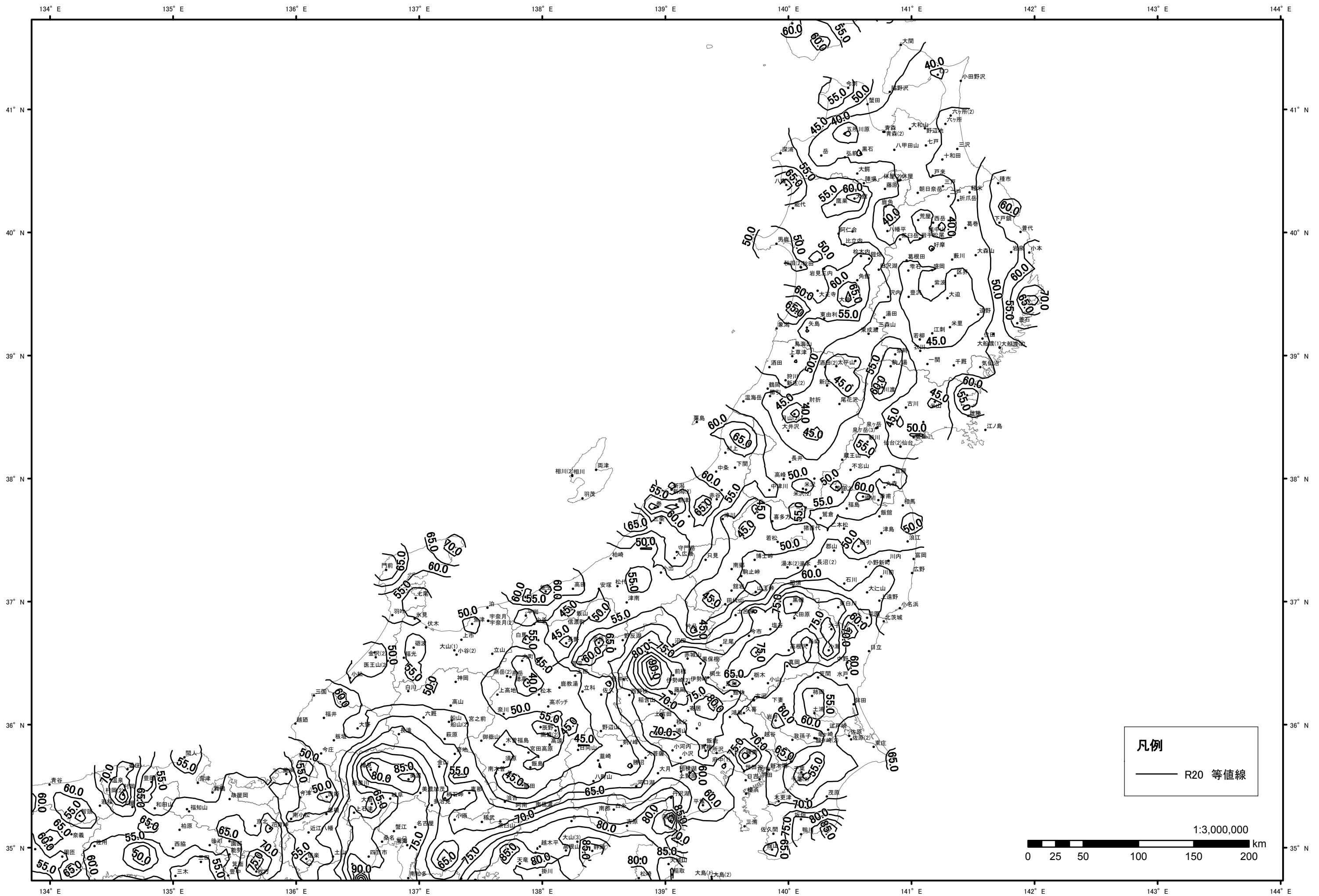
図 20年確率アメダス時間雨量 (R20) — 東北～関東～北陸
